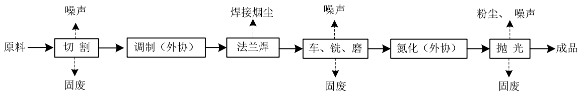
图 5-1 项目螺杆机筒生产工艺流程及产污环节图
