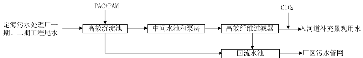
图 2-3 三期工程工艺流程图
