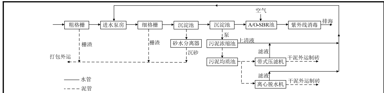
图 2-1 一期工程工艺流程图
