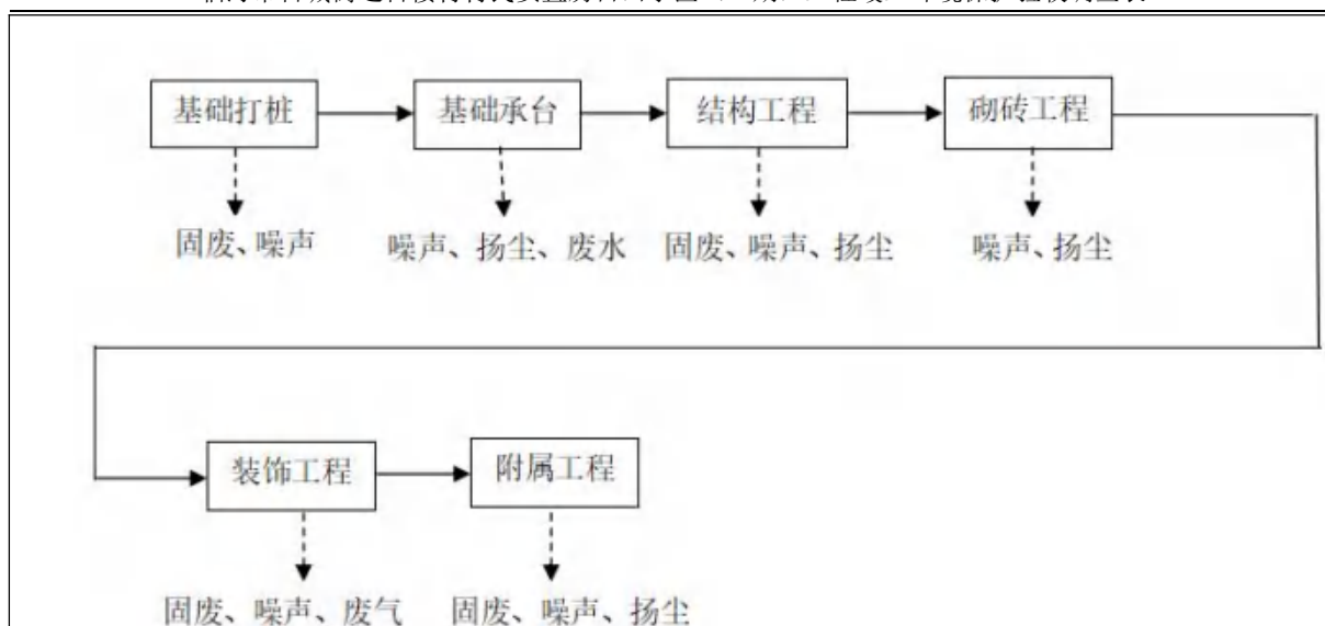
图 4-1 施工期工艺流程图
